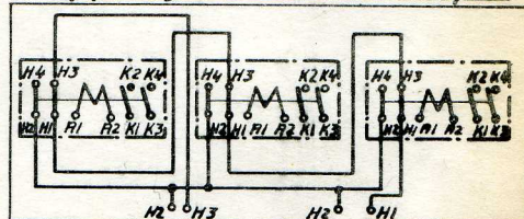
Kopplingsschema för M/40
