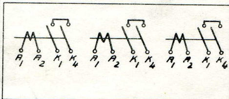
Kopplingsschema för M/37
